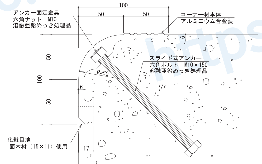
コーナー材取付け断面図 S = 1 : 2
