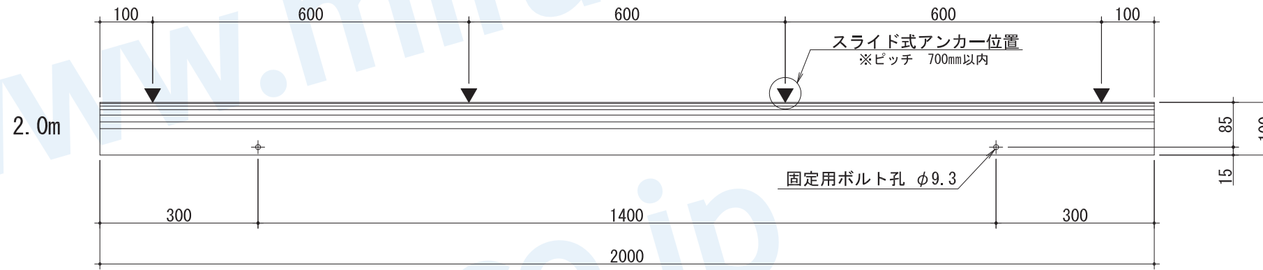
正面図 S = 1 : 10
