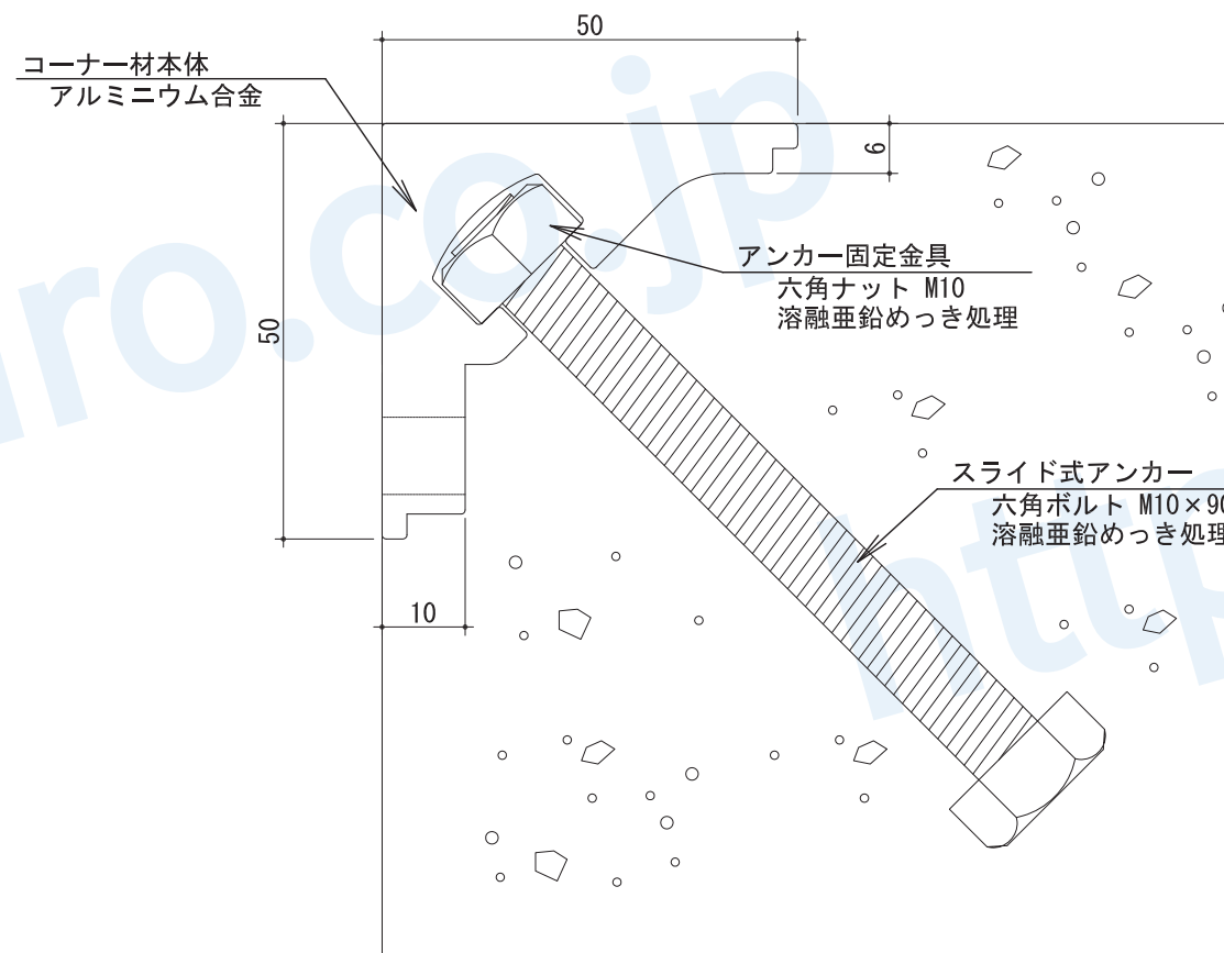
標準断面図 S = 1 : 1
