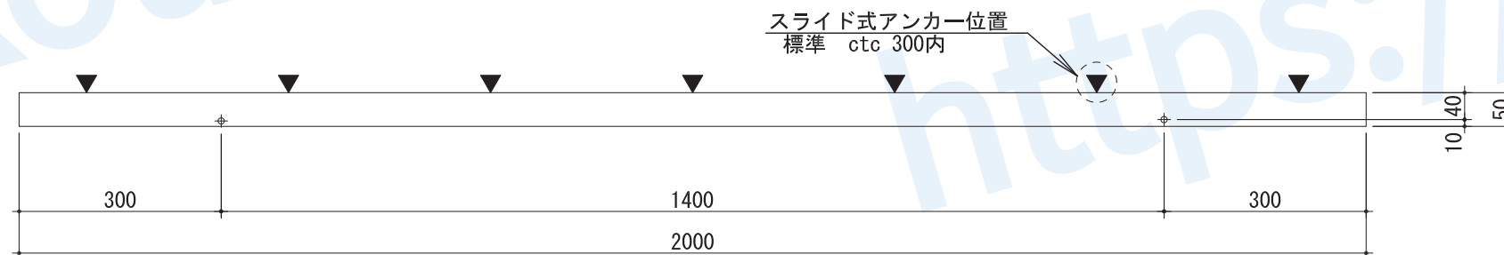
正面図 S = 1 : 10
